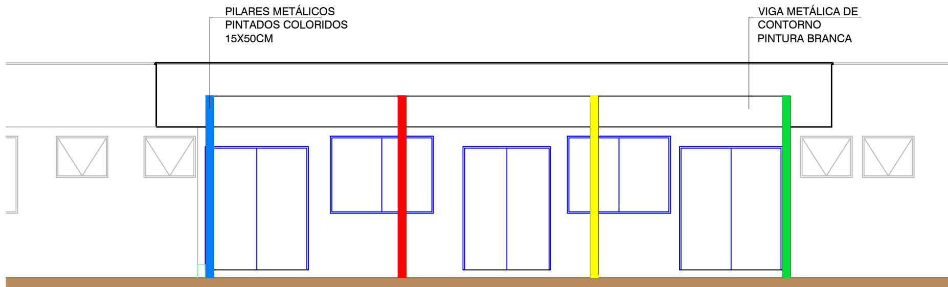
VISTA FRONTAL- ESC 1:75
