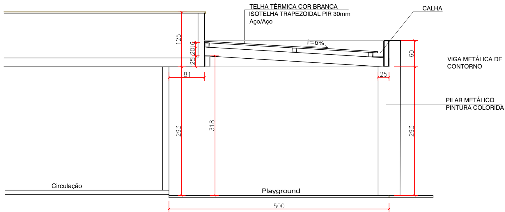
CORTE - ESC 1:50
