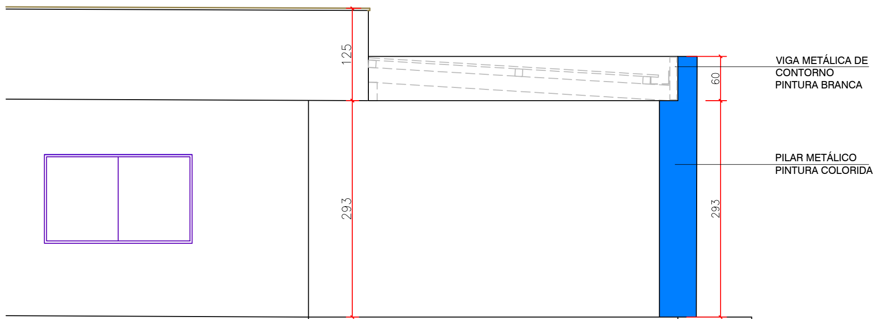
VISTA LATERAL- ESC 1:50
