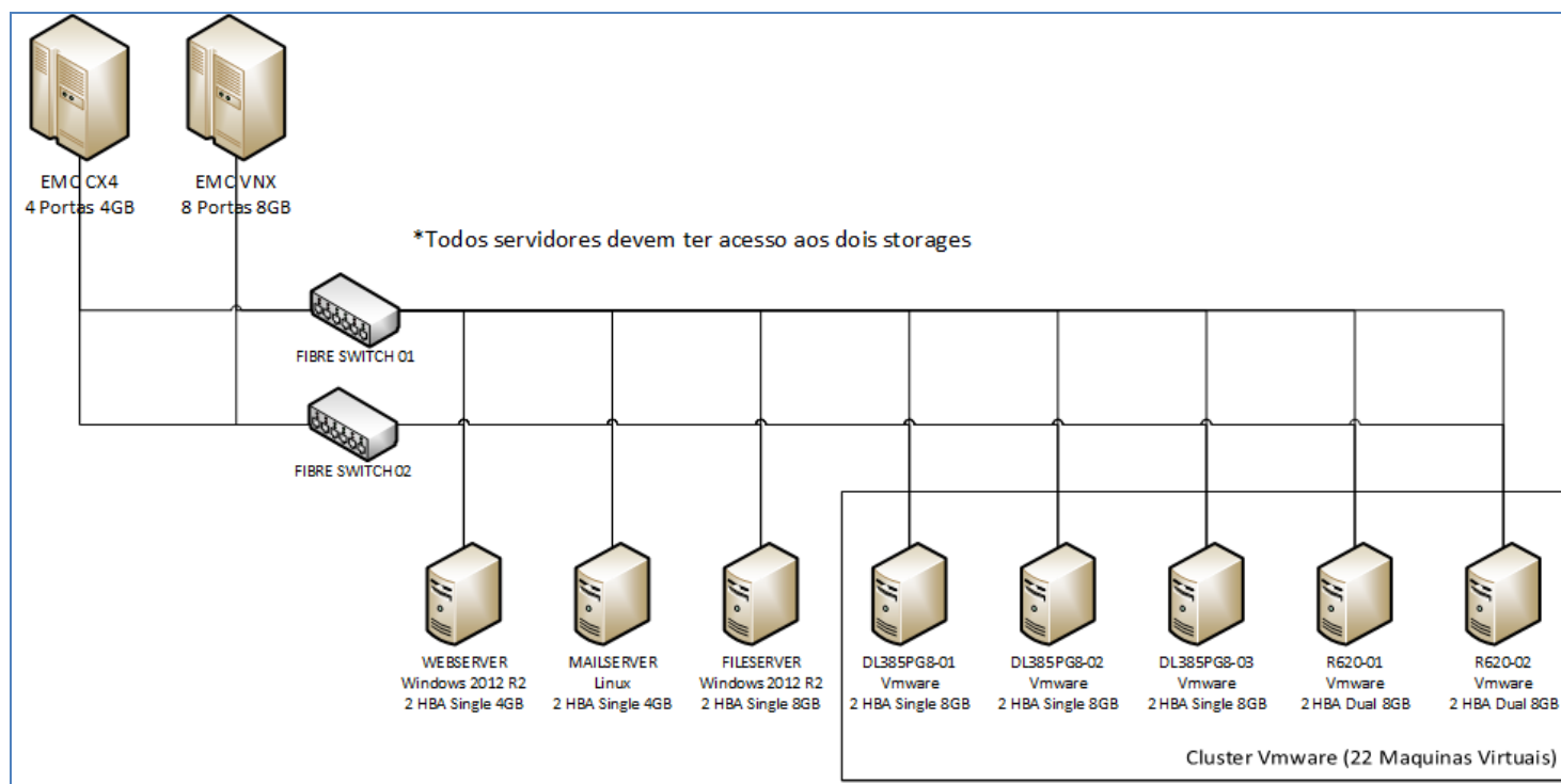
Figura 1: arquitetura da Rede SAN TCEGO
